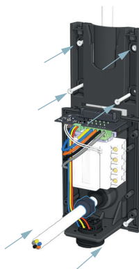
3. Przykręcenie tylnego panelu do ściany — dokręcenie wpustu kablowe
