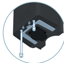
11. Montaż blendy
