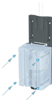
6. Montaż osłony za pomocą czterech śrub
