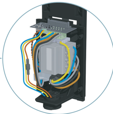
3. Przykręcenie tylnego panelu do ściany — dokręcenie wpustu kablowe
